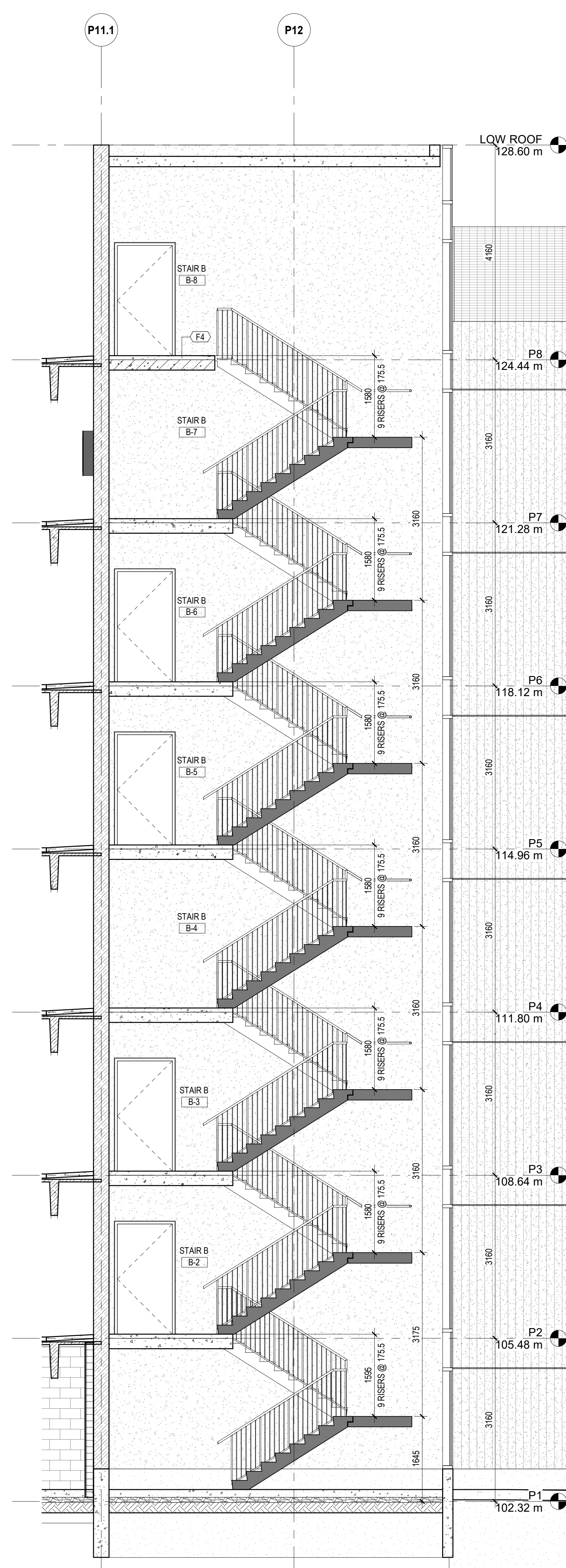
SECTION 1 - STAIR B SCALE: 1:50 A602
