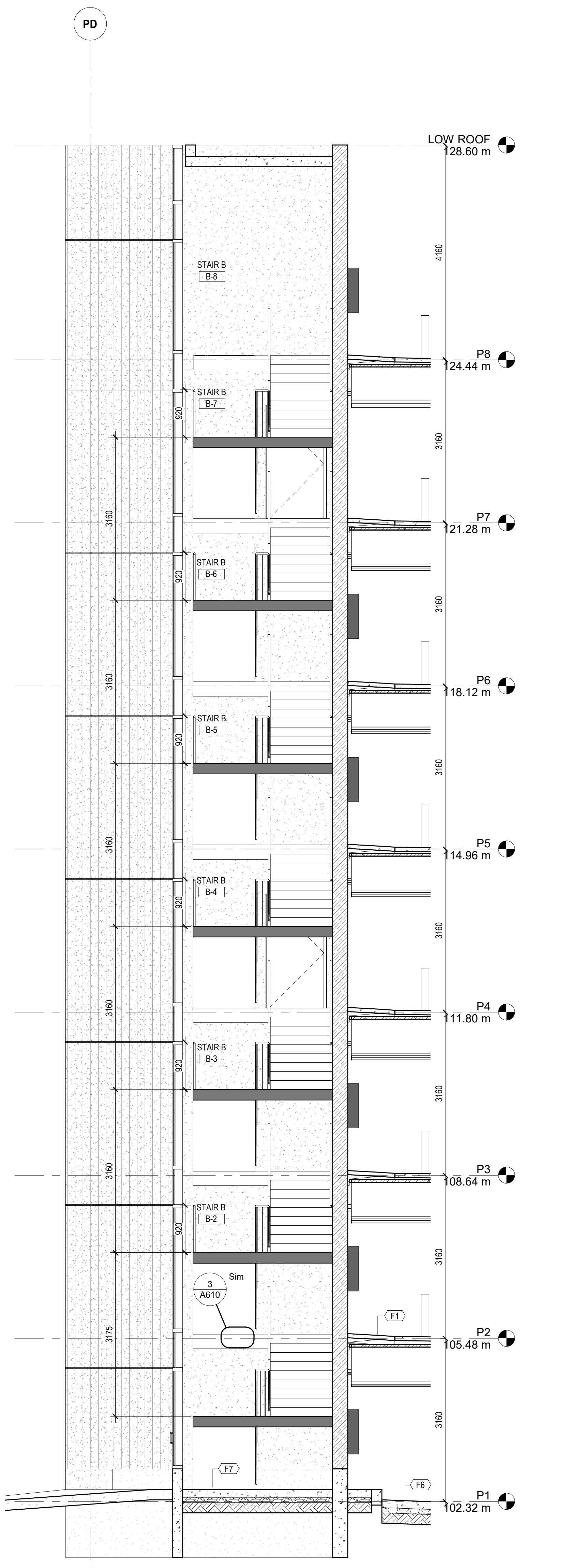
SECTION 2 - STAIR B SCALE: 1:50 A602
