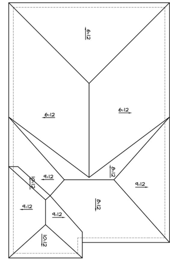
ROOF PLAN Scale: N.T.S.
