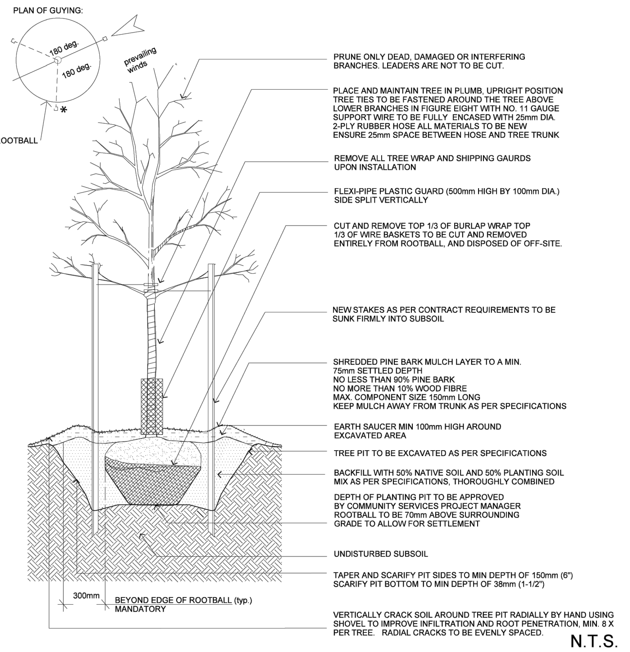
Detail: 02950-1
